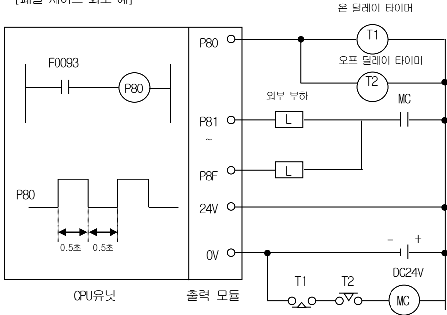
[페일 세이프 회로 예]
