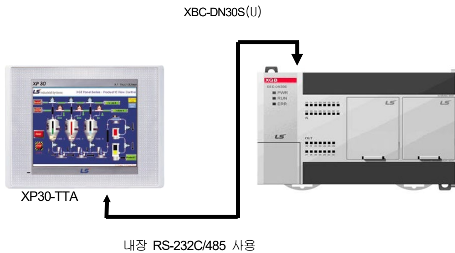
(d) 기본 유닛의 RS-232C/485 내장포트를 사용하여 모니터링 기기등과 1:1로 접속하여 사용하는 경우
