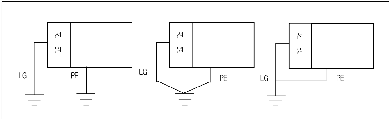
가) 전용접지: 가장 좋음 나) 공용접지: 양호 다) 공용접지: 불량
