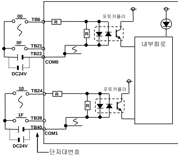
회로 구성
