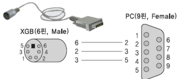
PMC-310S 결선도
