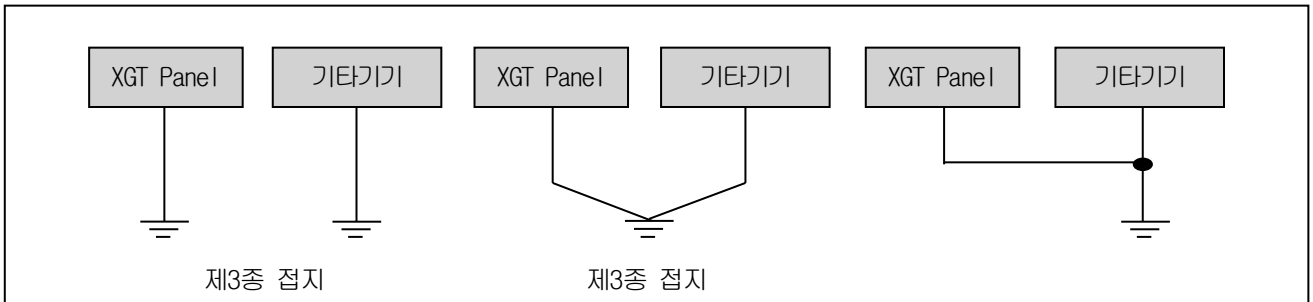
가) 전용접지: 가장 좋음
