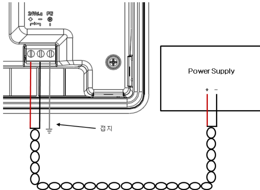
[ DC 전원 연결 ]
