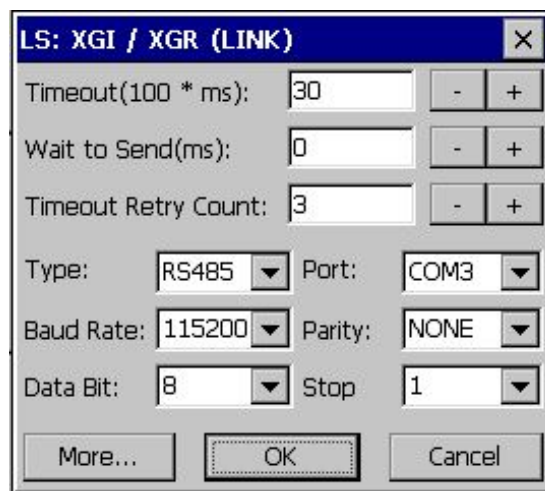
[PLC 통신 설정 화면]
