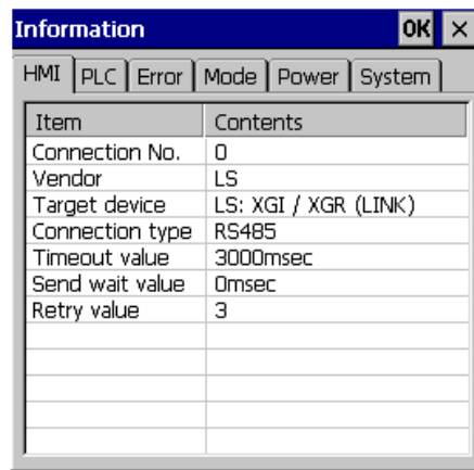
[PLC 연결 정보]
