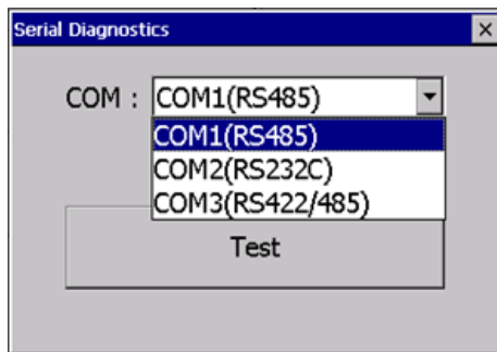
[시리얼 포트 선택 화면]
