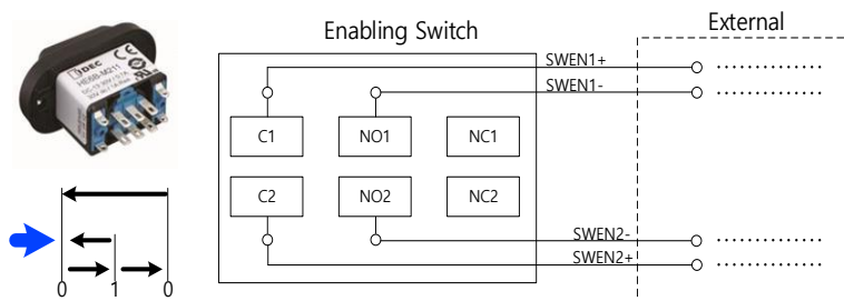
[그림 2.2.3] Enable Switch 구성
