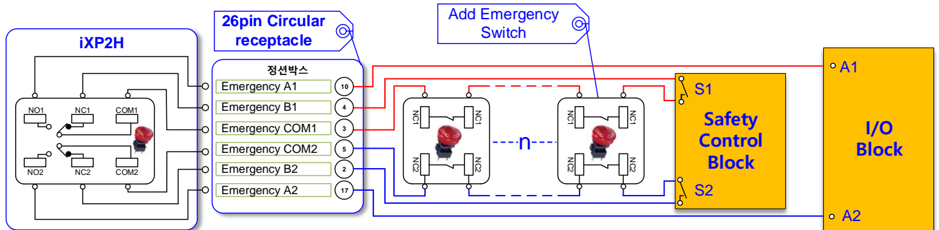
[Emergency Stop Switch 배선 예제]
