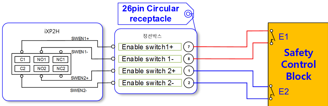
[Enabling Switch 배선 예제]
