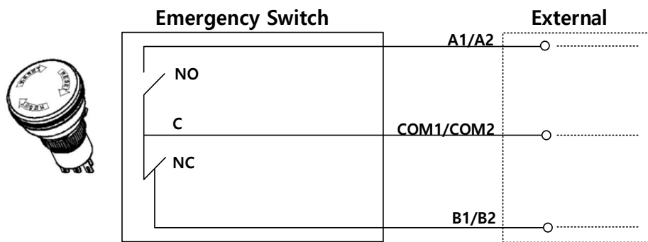
[그림 2.2.2] Emergency Stop Switch 구성
