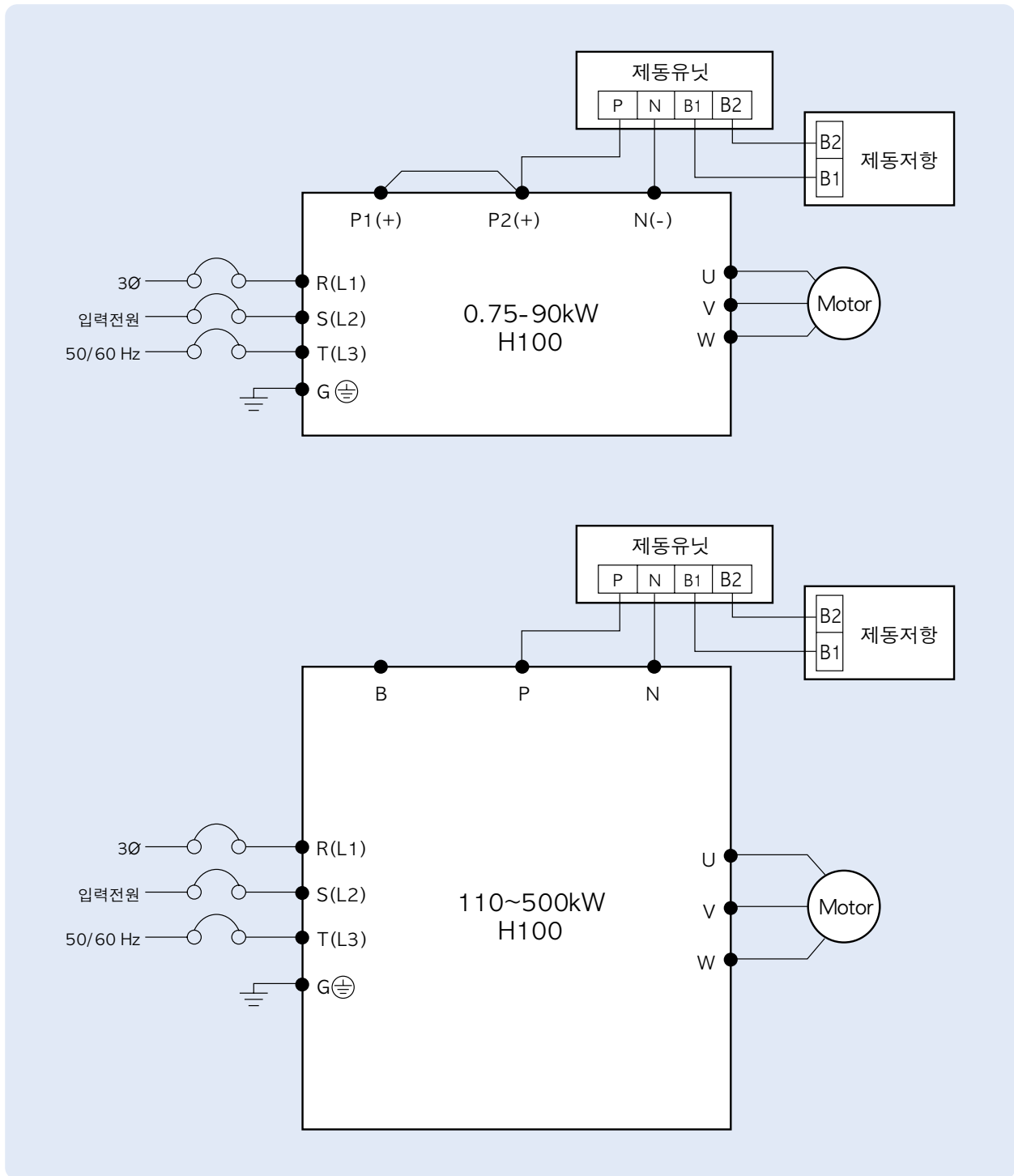
제동 유닛 및 제동저항 기본 결선도
