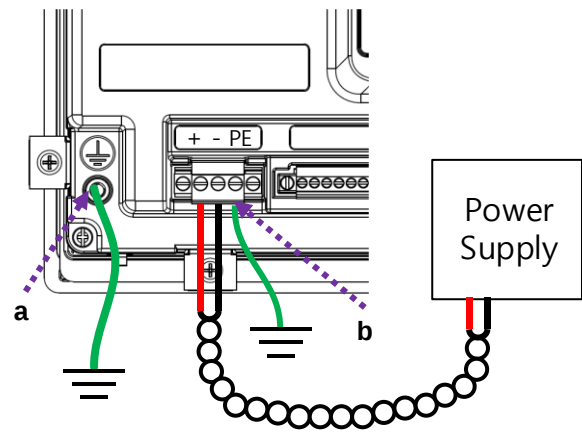
[DC 전원 연결]
