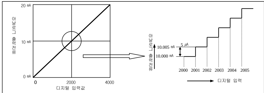
D/A 변환 특성 (전류 출력)
