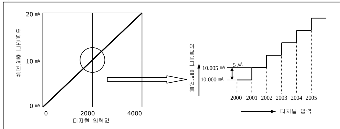
D/A 변환 특성 (전류 출력)
