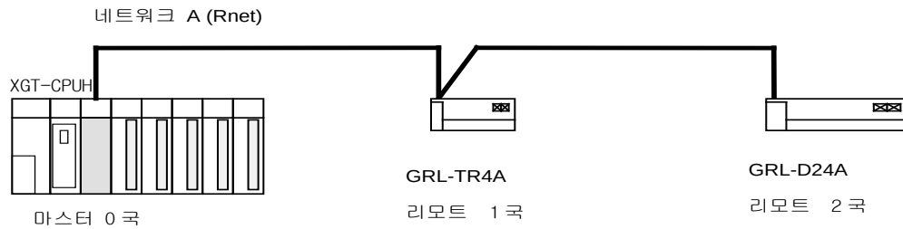
I/O 구성 및 송수신 흐름
