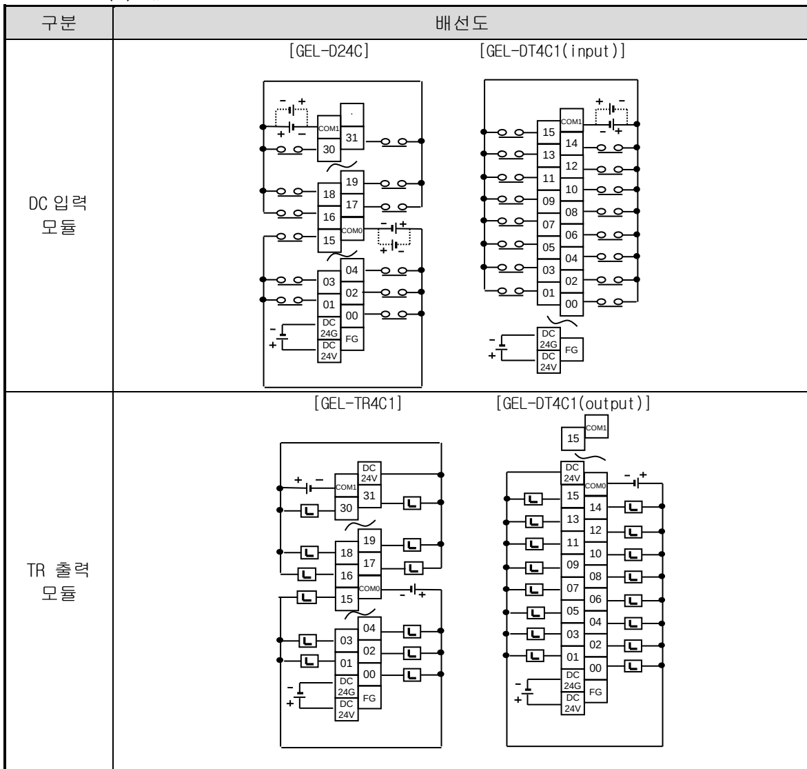
(2) 배선도
